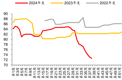
图 13: 光伏玻璃开工率 (%)
