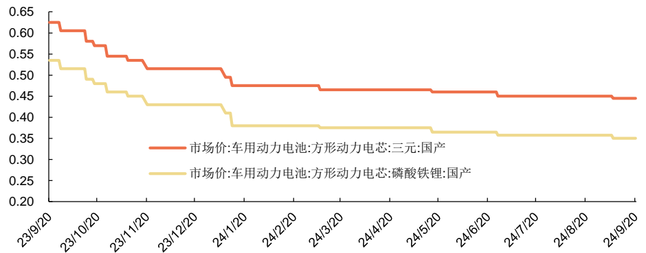
图8：车用动力电池价格（元/Wh）
