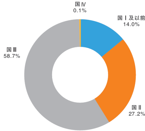
图表 26 按排放标准划分的工程机械 PM 排放量构成
