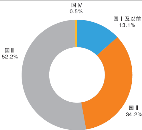
图表 24 按排放标准划分的工程机械 HC 排放量构成
