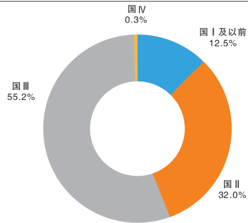
图表 25 按排放标准划分的工程机械 NOx 排放量构成
