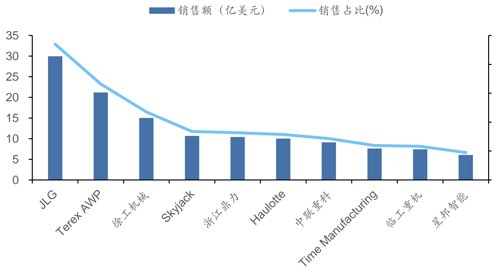
图表 40 2023 年主要企业高空作业平台设备销售额及占比
