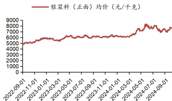
图表 38: 银浆料(正面)均价走势(元/千克)
