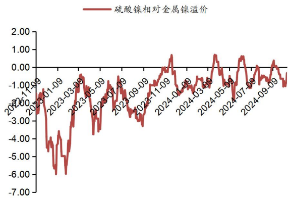
图表 19: 硫酸镍相对金属镍溢价走势 (万元/吨)
