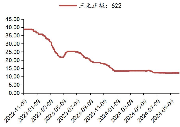
图表 31：三元正极 622 价格走势（万元/吨）
