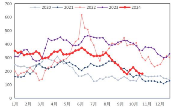
图 58: 石脑油、PX 价差 (美元/吨)
