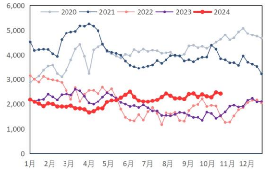
图 44: 原油、均聚聚丙烯价差 (元/吨, 元/吨)
