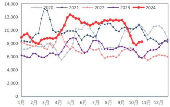
图 54: 原油、MMA 价差 (元/吨, 元/吨)
