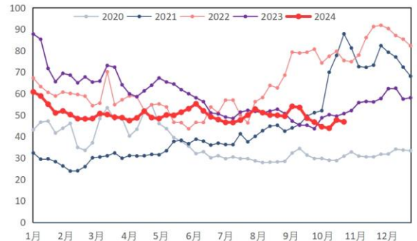
图 12: 原油、国内航煤价差 (美元/桶, 美元/桶)
