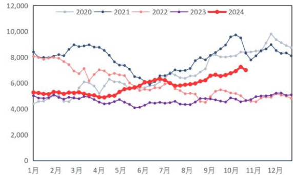
图 32: 原油、聚乙烯 LDPE 价差 (元/吨, 元/吨)
