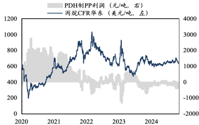
华东丙烷价格及PDH制PP盈利（美元/吨，元/吨）
