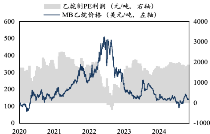
MB乙烷价格及乙烷裂解制PE盈利（美元/吨，元/吨）
