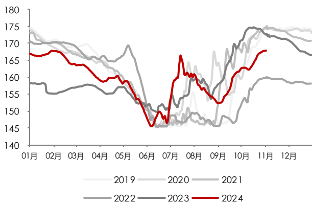
图表 5：24Q3 三峡水库水位为历年较低水平
