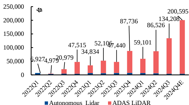
图 1、禾赛科技激光雷达出货量（含预测）
