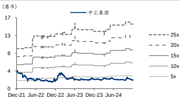
图表3: 中汇集团 PE-Bands
