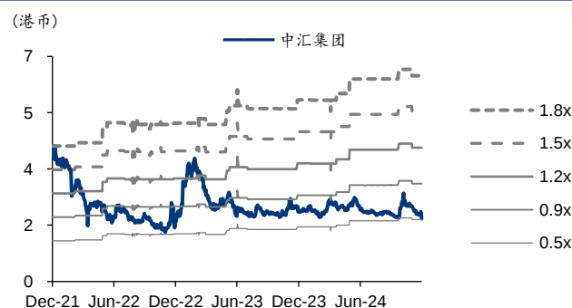
图表4: 中汇集团 PB-Bands
