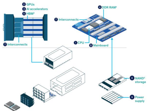
图 16: AI 服务器内部结构图
