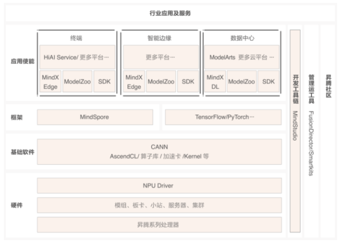
图 114：昇腾计算系统架构框图
