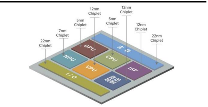
图 105: 基于 Chiplet 异构架构应用处理器的示意图
