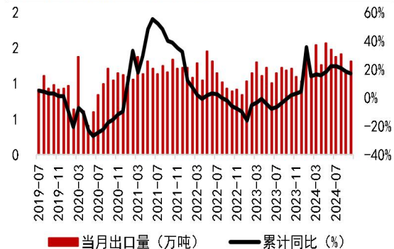
图：中国涤纶帘子布出口量
