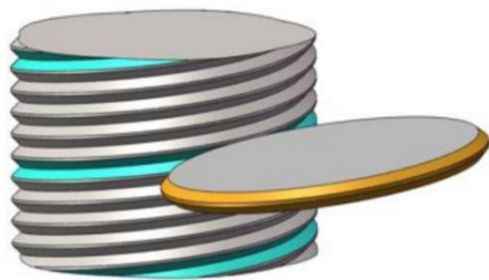
图34: 砂轮磨削加工外螺纹螺旋面
