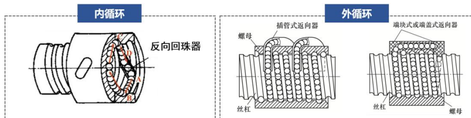
图18: 内循环式与外循环式滚珠丝杠
