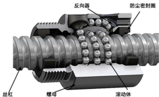
图14：滚珠丝杠结构
