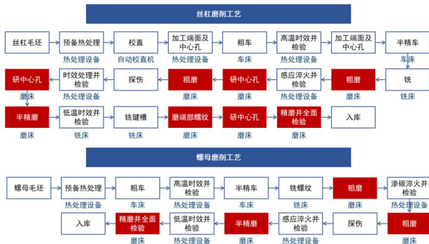
图37: 行星滚柱丝杠的磨削加工工艺流程
