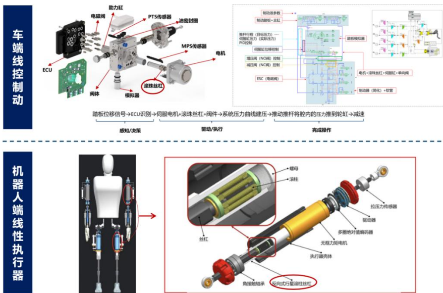
图3：汽车与人形机器人的线控制动核心部件拆解
