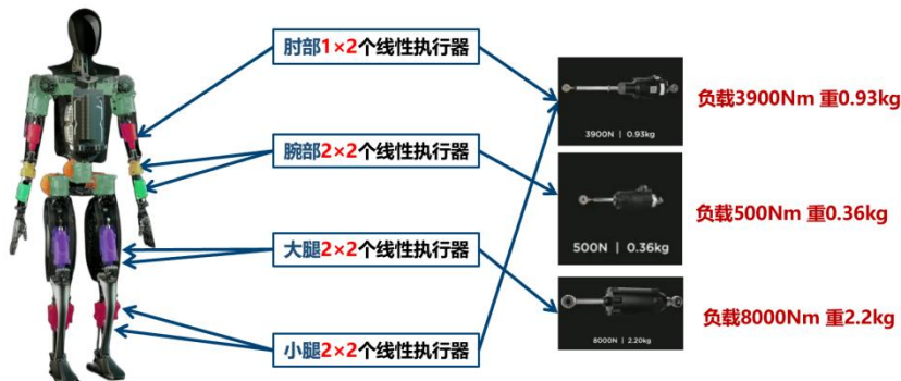
图56: 特斯拉 Optimus 机器人丝杠方案
