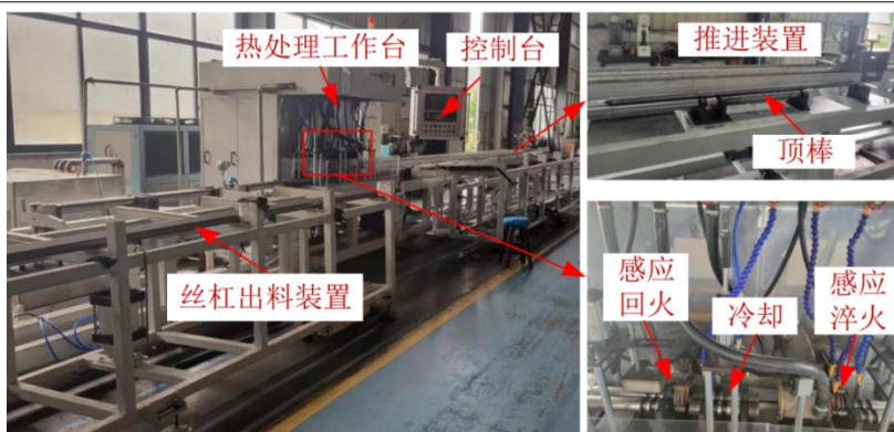
图45: 热处理设备
