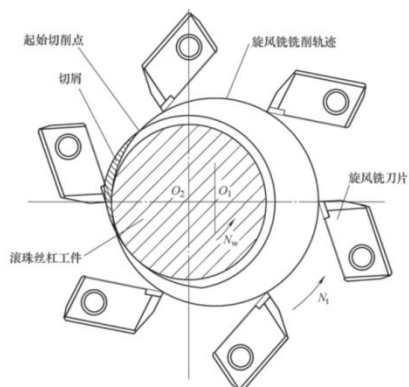
图38: 旋风硬铣削加工原理图
