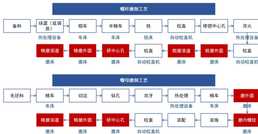
图36: 滚珠丝杠的磨削加工工艺流程
