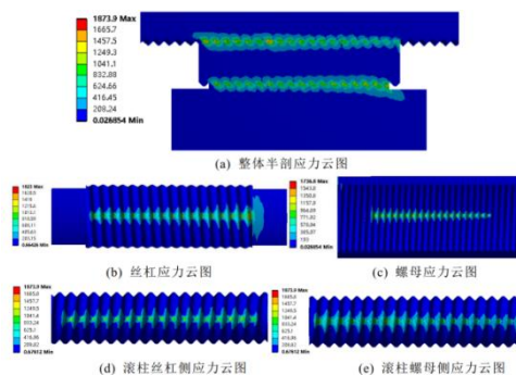
图24：行星滚柱丝杠多个滚柱共同承受载荷
