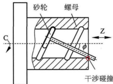
图35: 砂轮磨削加工螺母内螺纹
