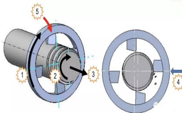
图39: 旋风铣五大加工运动
