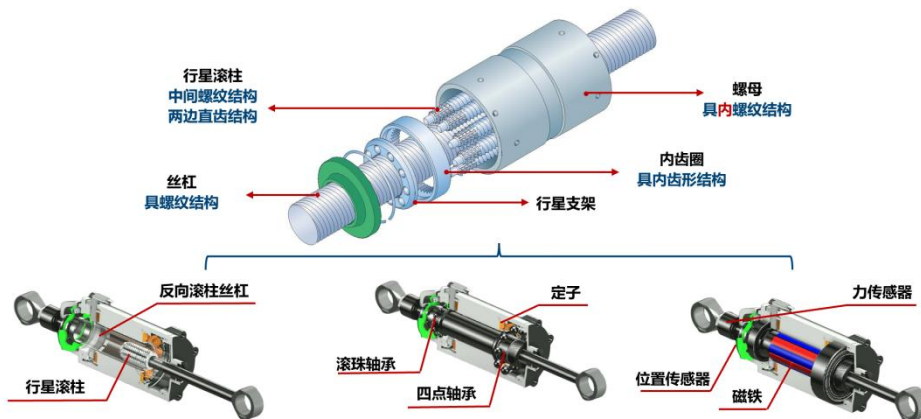
图9：行星滚柱丝杠及相关构造拆解
