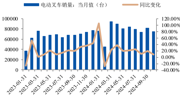
图 18：电动叉车当月销量及增速
