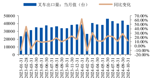
图 15：叉车当月出口量及增速
