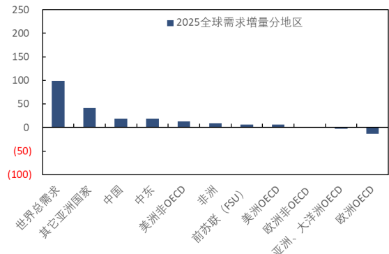
图 79: 2024.11 IEA 预测 2025 年全球原油分地区需求增量 (万桶/日)
