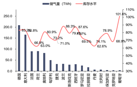
图 34：欧盟各国储气量及库存水平（2024/12/20，TWh）
