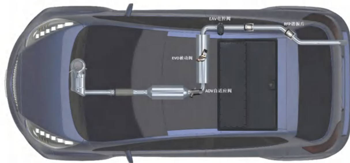
佛吉亚混动新能源汽车的排气系统整体解决方案
