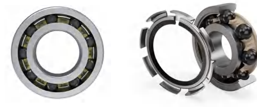
斯凯孚混合陶瓷球轴承与导电环
