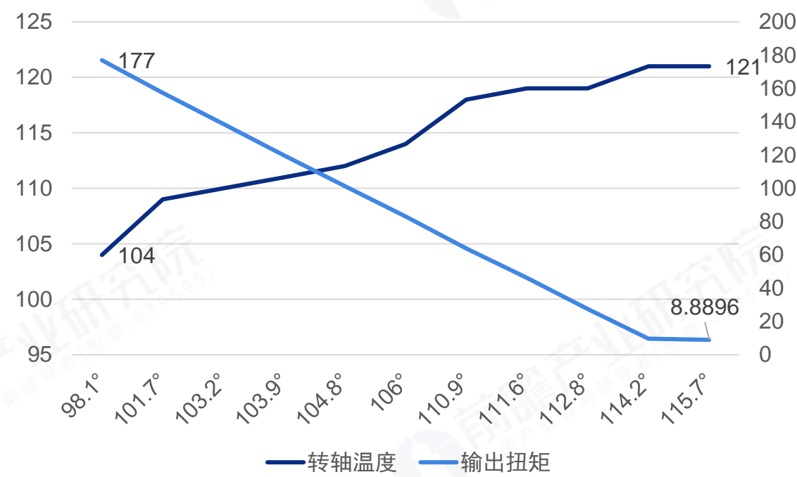
温升对电机性能的影响（单位：°C，nm）
