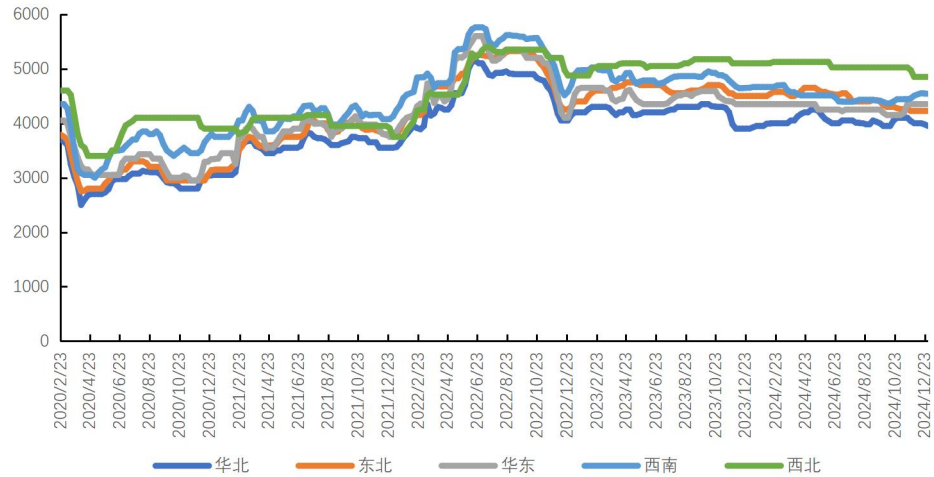
图表 18：2020 年至今各地区 SBS 改性沥青价格走势（单位：元/吨）
