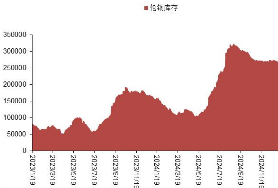
图表 9: LME 铜库存 (吨)
