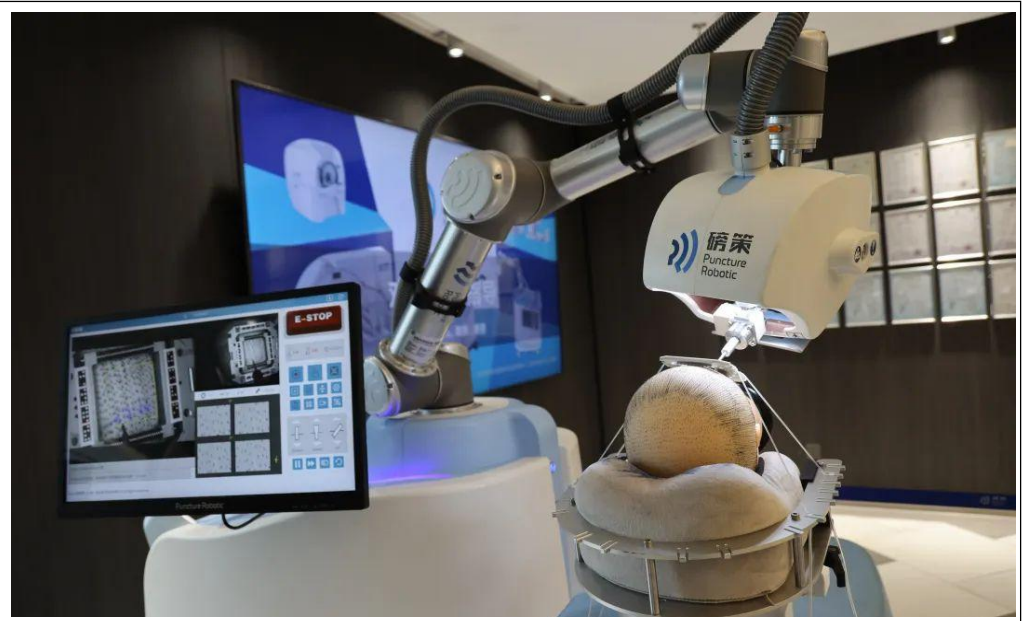
图 4：HAIRO®植发机器人
