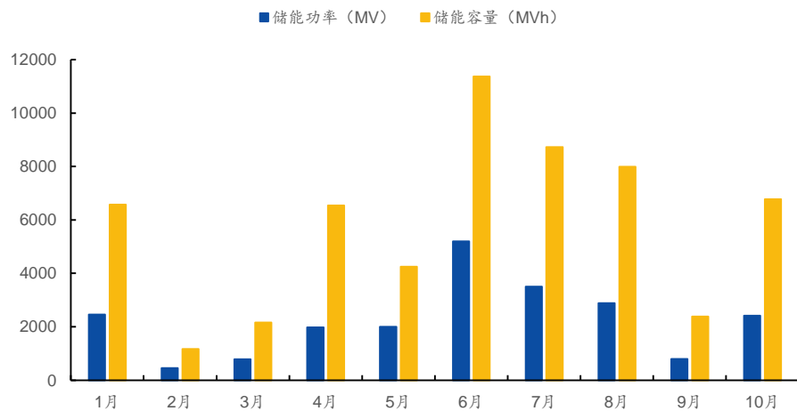
图 18：2024 年国内新型储能新增装机情况
