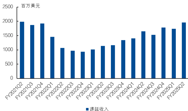
图3、递延收入
