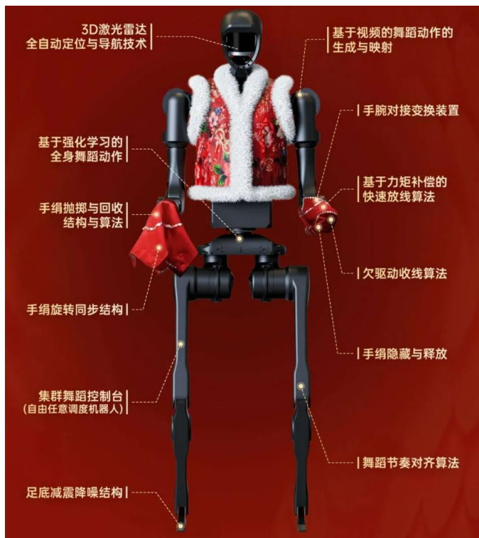
图表：宇树机器人春晚舞蹈主要技术解析
