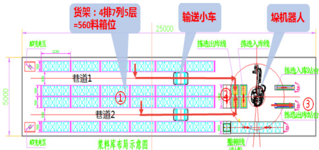
图 风华高科浆料出入库管理流程
