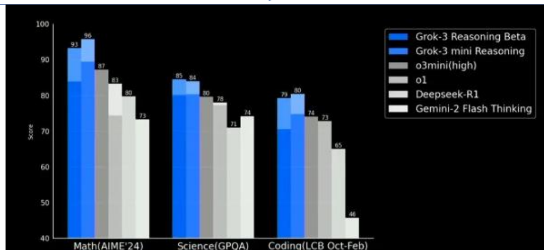
图37：Grok-3的推理性能得分领先于o3mini和DeepSeek-R1
