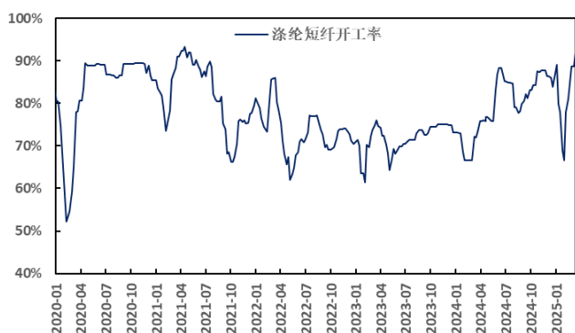
图 80: 2020-2024 年涤纶短纤开工率 (%)
