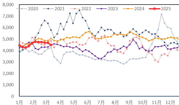
图 42: 原油、苯乙烯价差 (元/吨, 元/吨)
