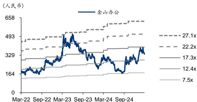
图表3: 金山办公 PB-Bands
