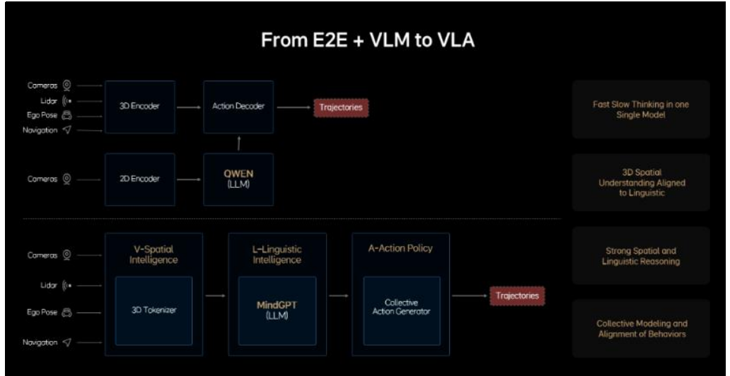
图8: MindVLA 将模型中所有模块进行了重新设计
