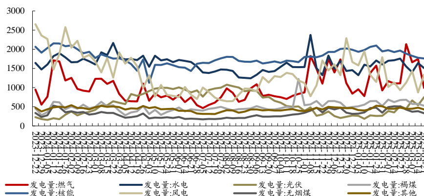
图7: 最近一年欧洲发电结构 (吉瓦时/日, 周度数据, 截至 2025/3/21)
