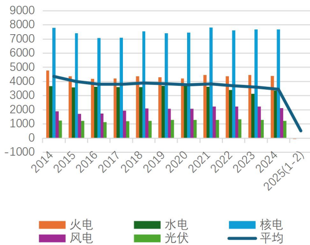
图 11：全国发电设备累计平均利用小时（小时）
