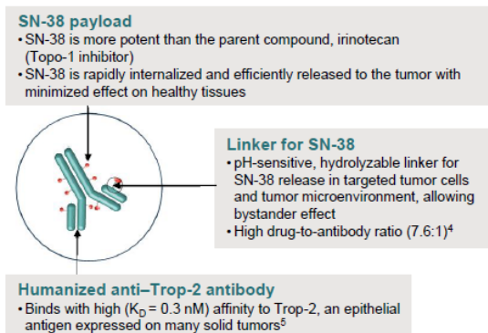
图61: Trodelvy 分子结构
