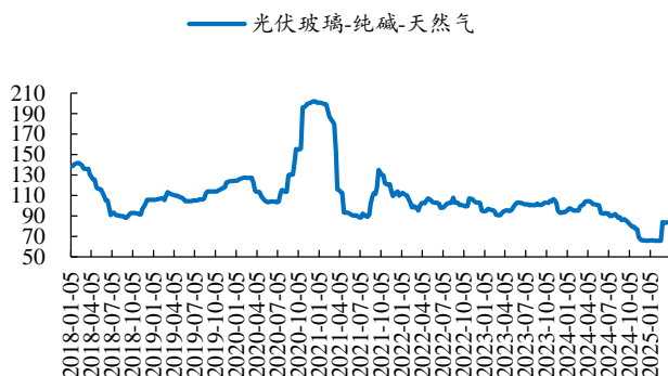
图51：光伏玻璃盈利环比上涨0.13%（元/重量箱）
