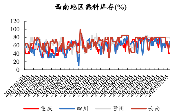
图21：本周西南地区熟料库存重庆、四川、贵州、云南环比持平
