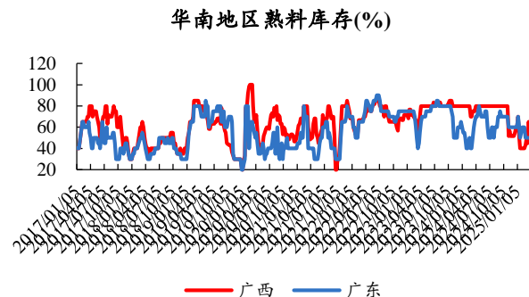
图17：本周华南地区熟料库存广东环比持平，广西环比下降
