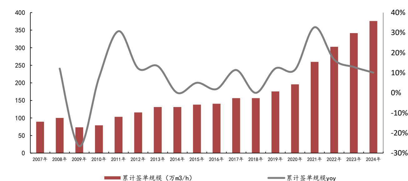
图3：公司管道气累计签单情况，构筑公司“防御”属性，公司未来管道气量的投放稳健增长
