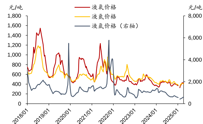
图1：2018年至今氧、氮、氩价格走势（元/吨）
