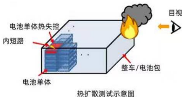
图1：热扩散测试示意图
