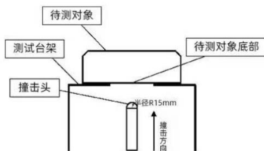
图2：底部撞击测试考察电池底部受到撞击后的防护能力
