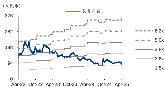
图表4: 长春高新 PB-Bands
