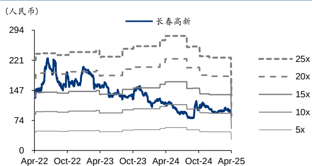
图表3: 长春高新 PE-Bands
