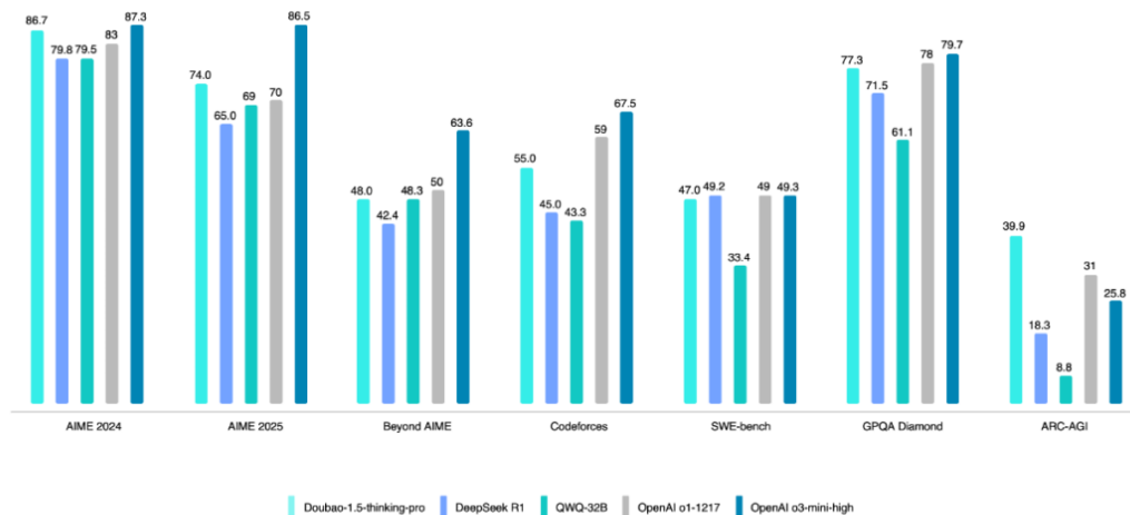
图表 2：豆包 1.5·深度思考模型，推理能力跻身全球第一梯队
