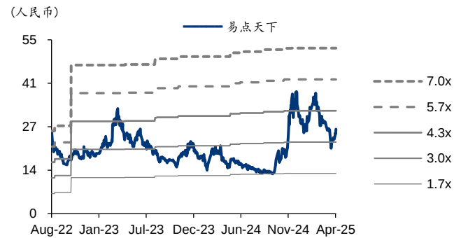
图表3: 易点天下 PB-Bands
