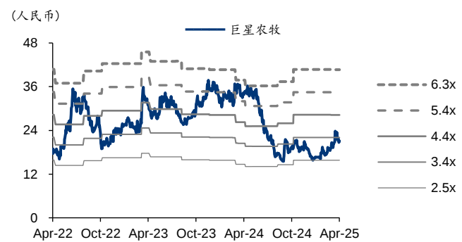
图表3：巨星农牧 PB-Bands
