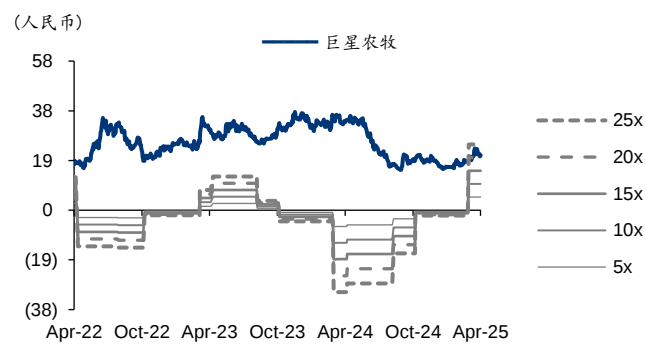
图表2：巨星农牧 PE-Bands
