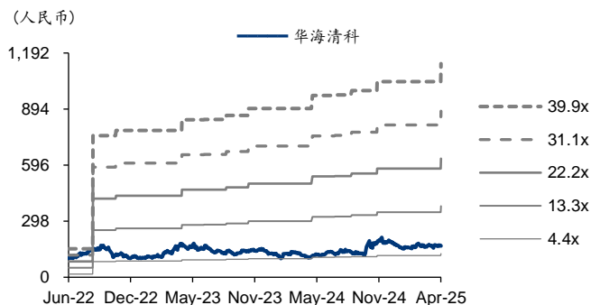
图表3: 华海清科 PB-Bands
