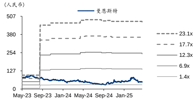
图表3：曼恩斯特 PB-Bands
