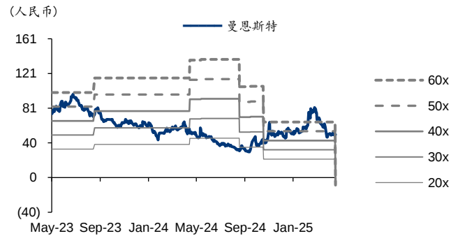
图表2：曼恩斯特 PE-Bands
