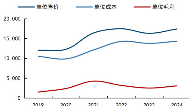
图4：电解铝盈利变化（元/吨）
