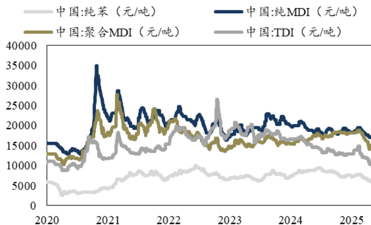
纯苯、纯MDI、聚合MDI、TDI价格走势（元/吨）
