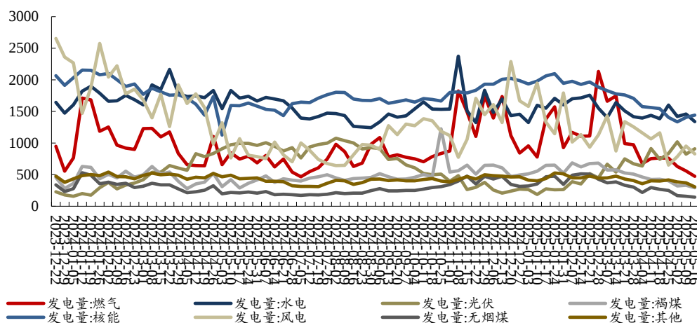
图7：最近一年欧洲发电结构（吉瓦时/日，周度数据，截至 2025/5/16）
