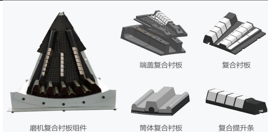
图29:公司磨机复合衬板（橡胶+耐磨合金）
