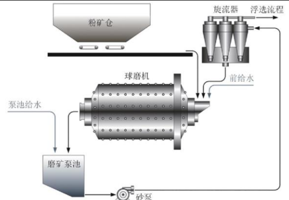
图28:球磨机在磨矿过程中的应用
