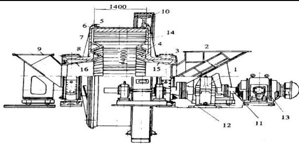
图 9-1 \phi 4000 \times 1400 干式自磨机构造
