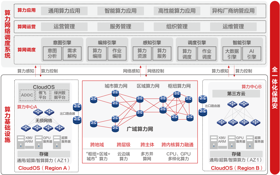
算力网络架构图
