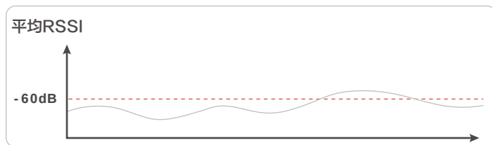
信号差算法
