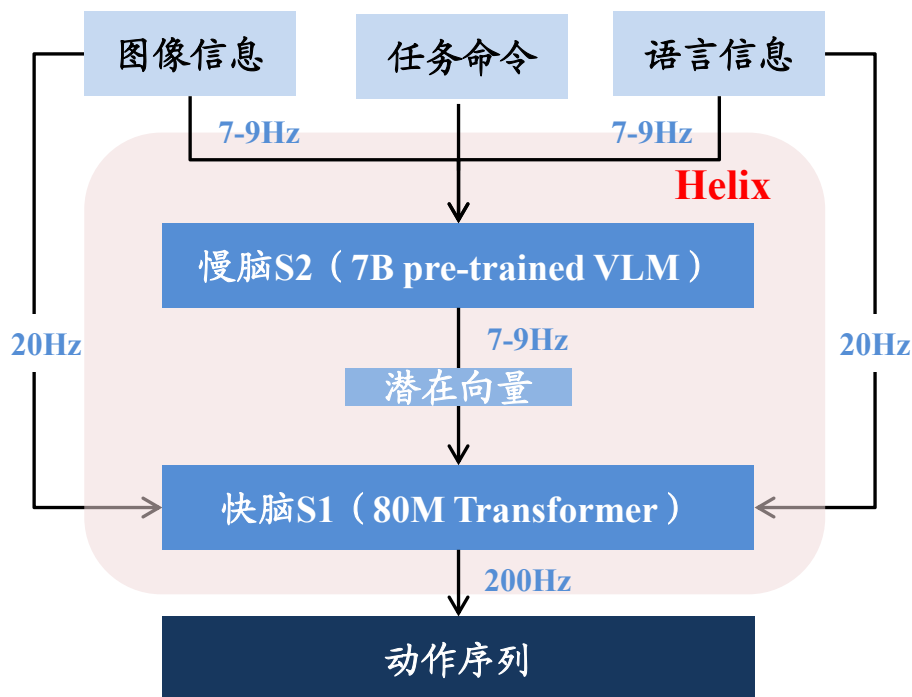
图：Helix模型架构
