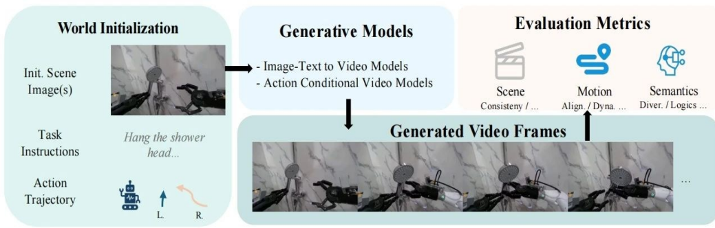
图：具身世界模型评测基准EWMBench
