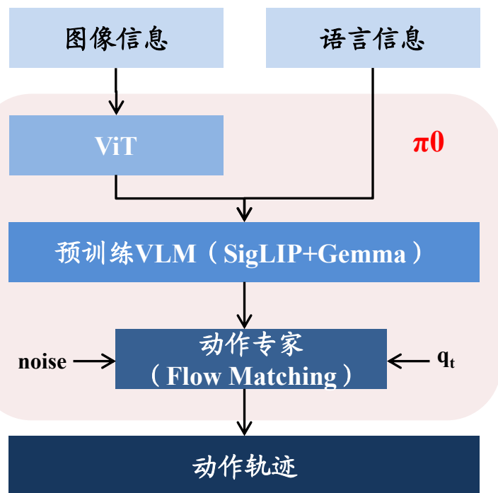
图: \pi 0 模型架构
