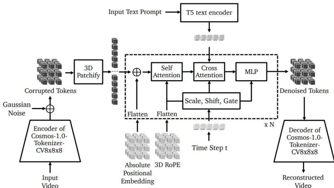
图：Cosmos-1.0-Diffusion WFM 的整体架构
