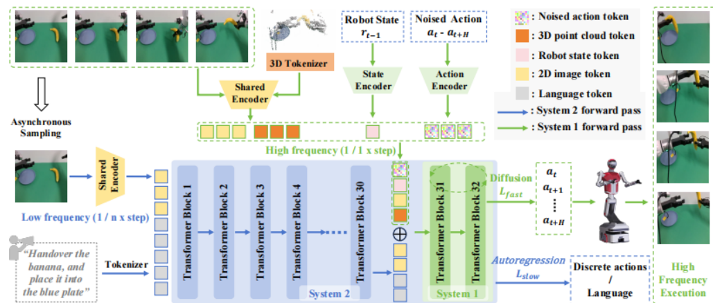
图：Fis-VLA模型架构
