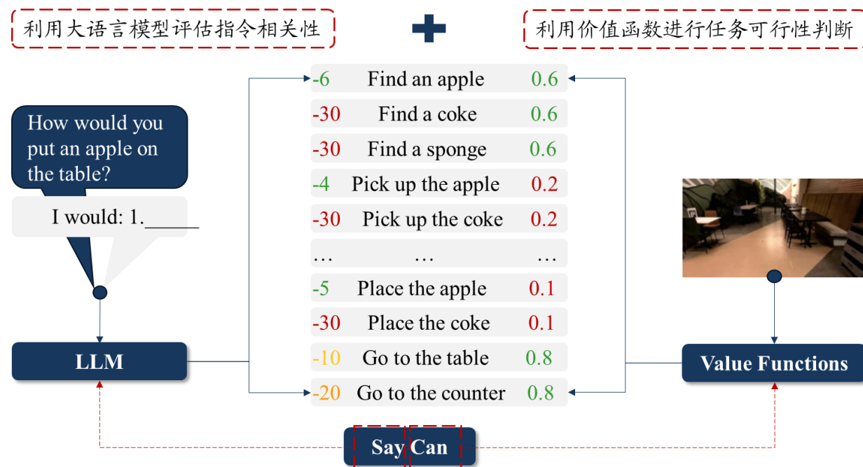
图：SayCan模型架构
