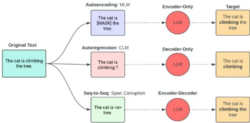
图：预训练策略图
