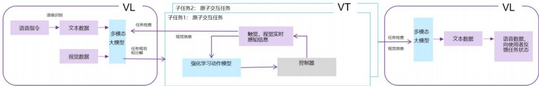
图：VTLA模型的构架原理
