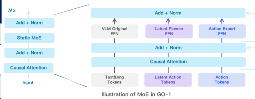
图：GO-1中的混合专家系统
