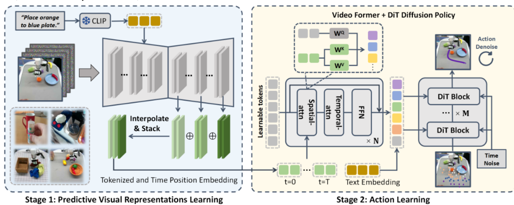
图：VPP学习框架
