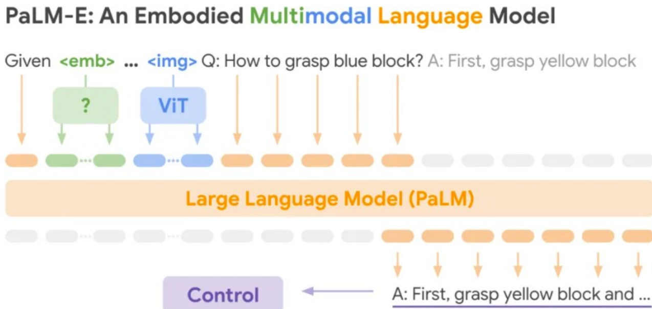
图：PaLM-E模型架构
