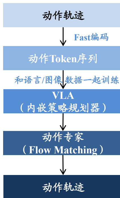
图: \pi 0.5 采用VLA
