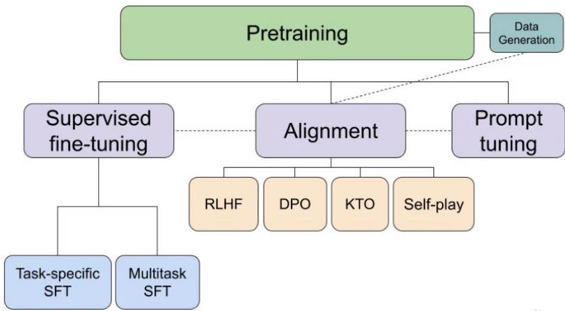
图：后训练流程图
