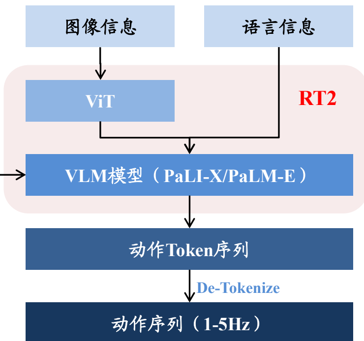
图：RT2模型架构
