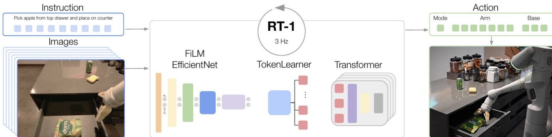
图：RT-1模型架构
