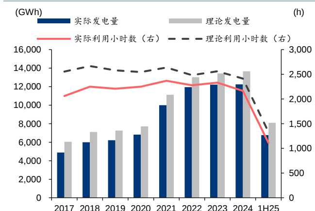
图表5: 节能风电 2017 年至 1H25 实际/理论发电量与小时数
