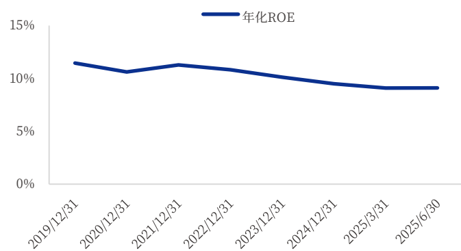
图2：中国银行 ROE
