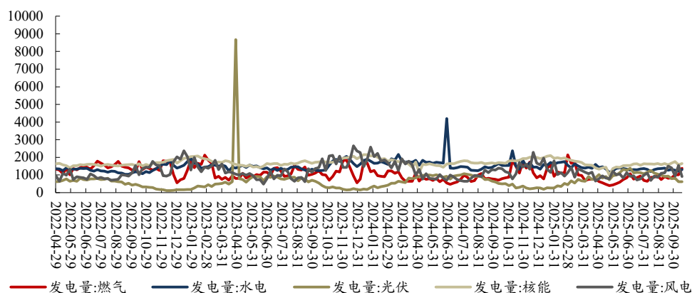
图7：最近一年欧洲发电结构（GWh/日，周度数据，截至 2025/10/17）
