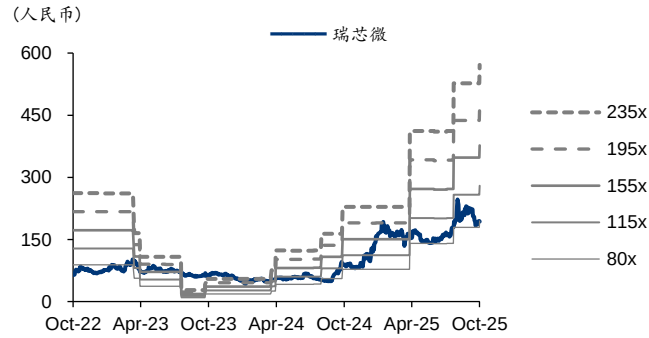
图表2：瑞芯微 PE-Bands
