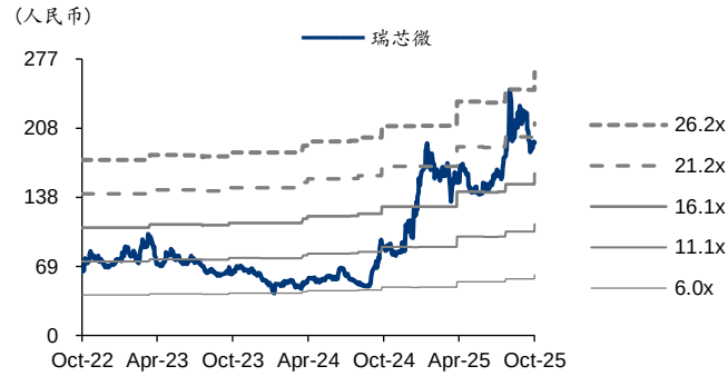
图表3：瑞芯微 PB-Bands
